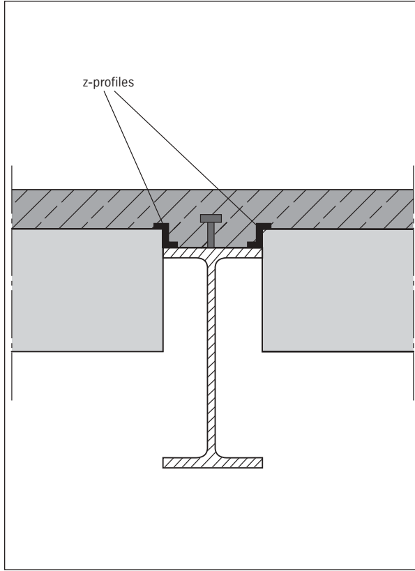
Edge formation
