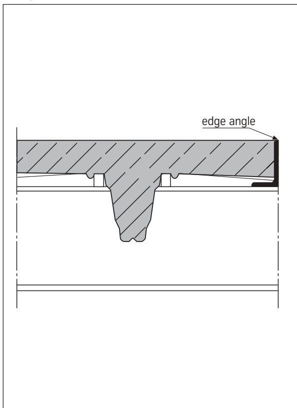
Edge formation
